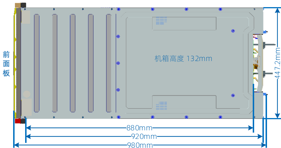
图 3-9 3U 扩展柜尺寸（俯视图）
