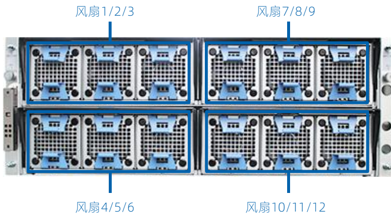
图 2-12 风扇模块
