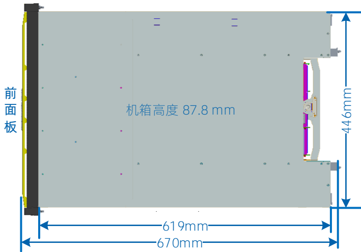
图 3-8 2U 扩展柜尺寸（俯视图）
