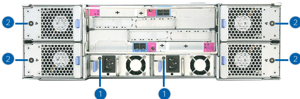
图 4-16 3U 扩展柜电源/风扇指示灯
