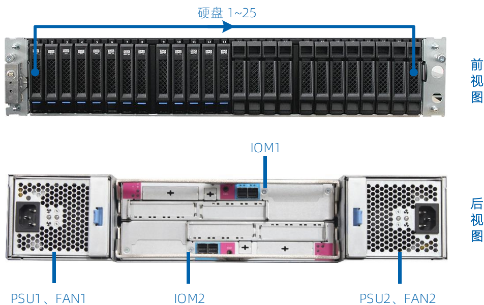
图 3-2 2U25 盘位扩展柜前后视图
