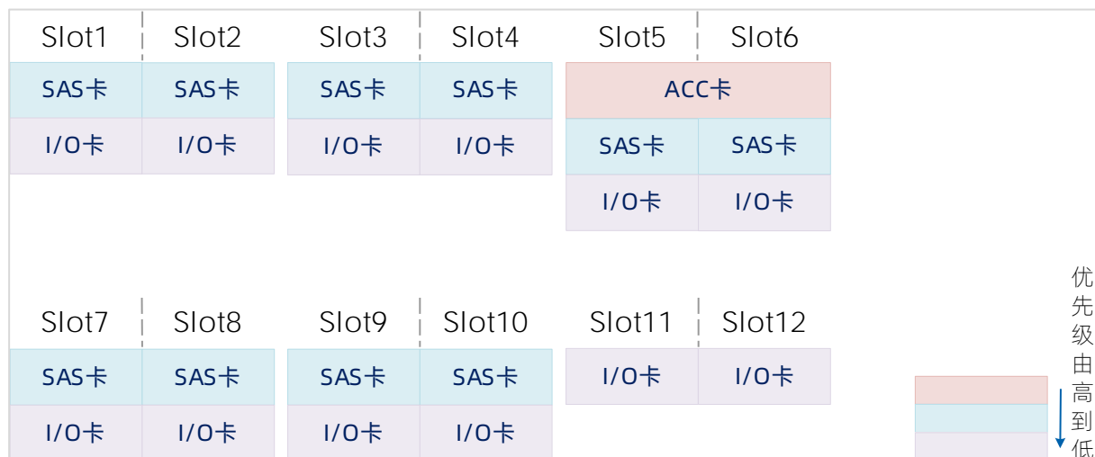
图 2-9 PCIe 插槽优先使用顺序
