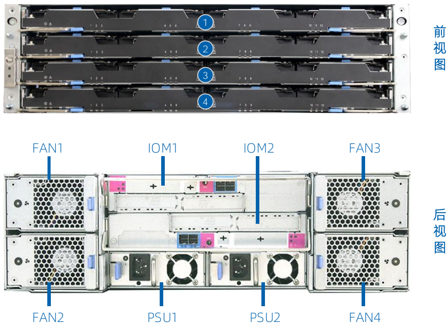
图 3-3 3U 扩展柜前后视图
