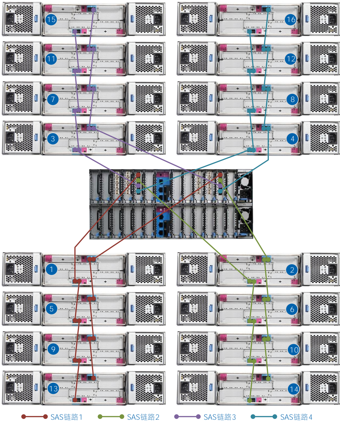
图 5-3 连接 16 台扩展柜（每控 1 张 4 口 SAS 卡）
