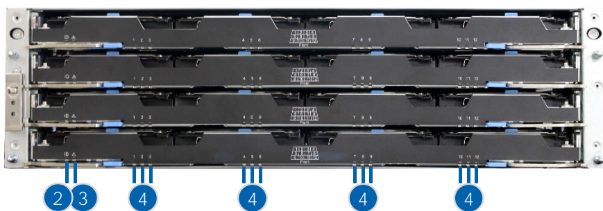
图 4-9 3U 扩展柜硬盘抽屉面板指示灯
