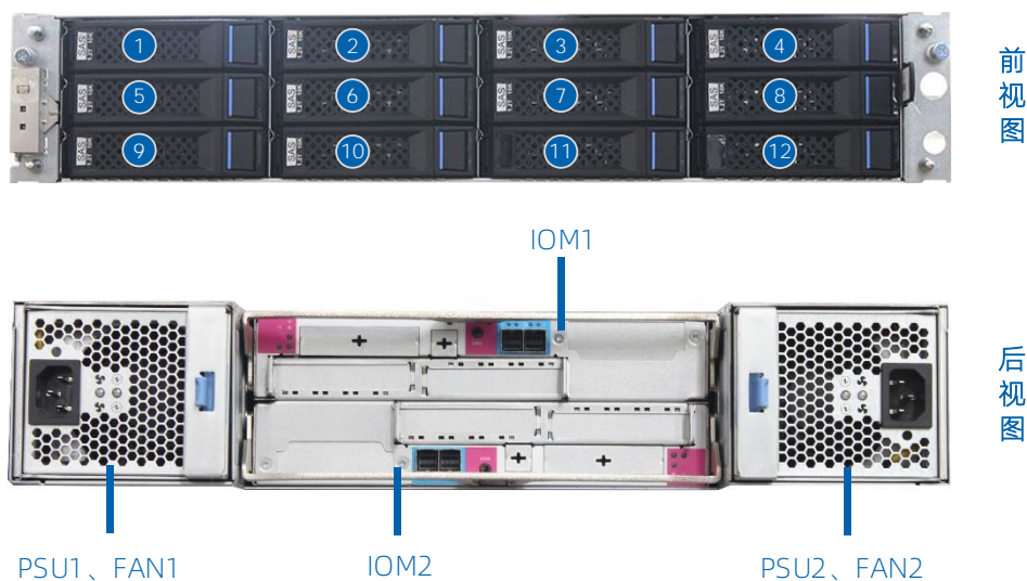
图 3-1 2U12 盘位扩展柜前后视图
