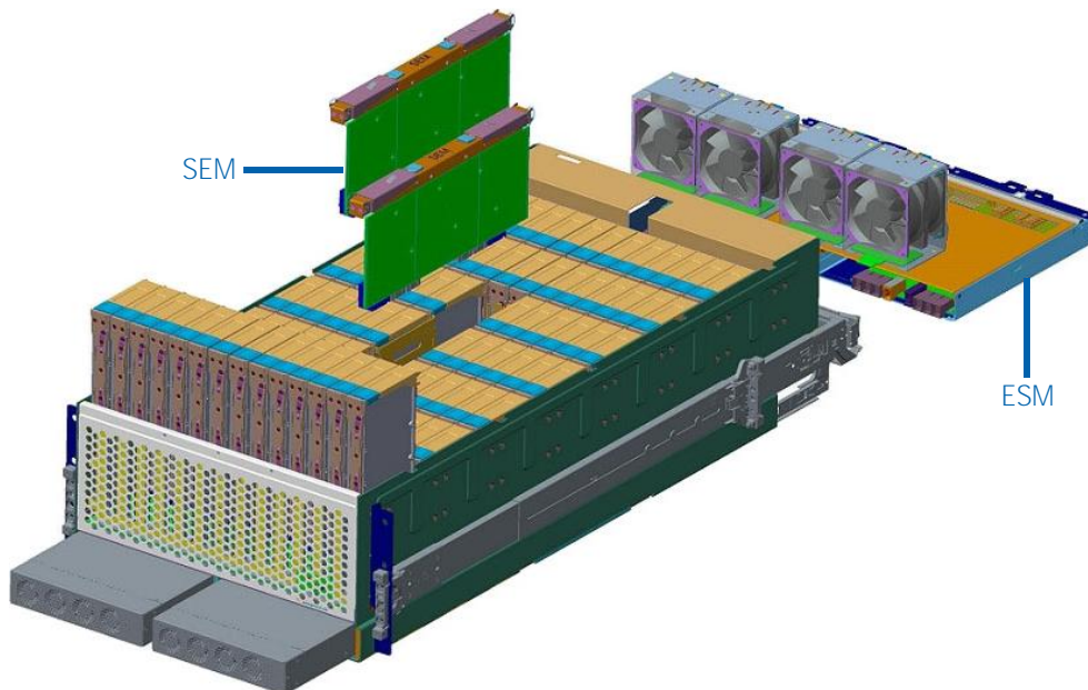
图 3-12 SEM 和 ESM 模块位置
