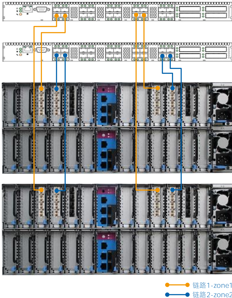
图 5-1 四个控制器冗余连接方式
