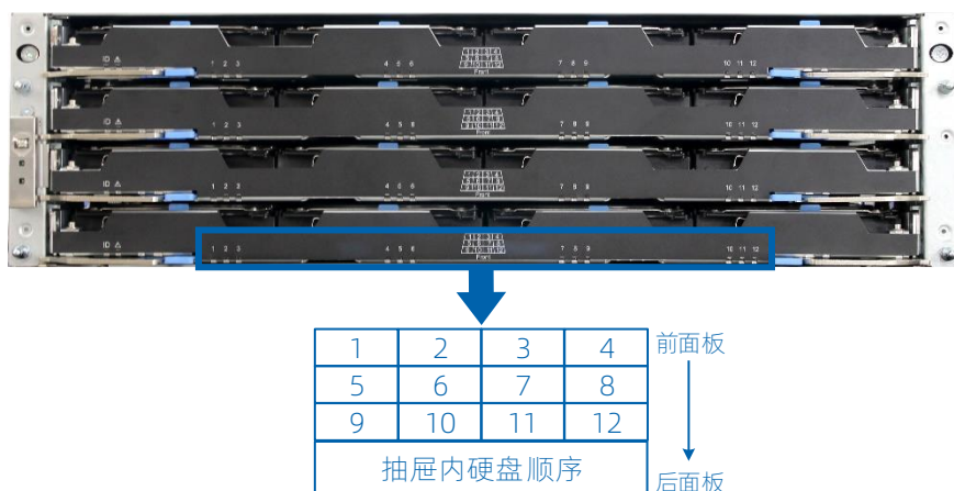
图 4-10 硬盘和硬盘指示灯的对应关系
