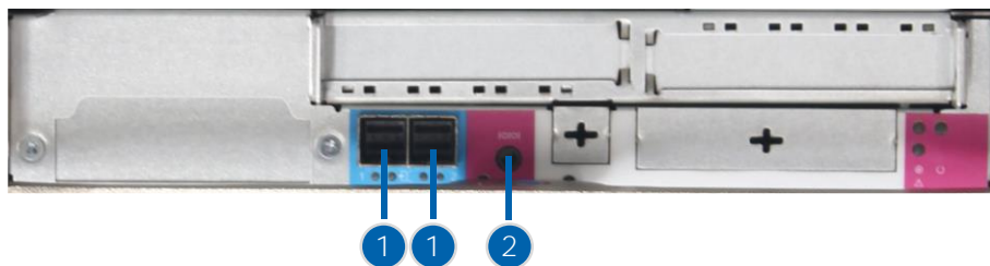
图 3-11 2U/3U 扩展柜 IO 模块后视图
