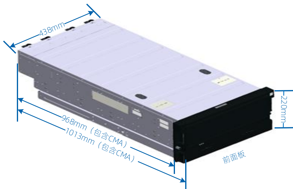
图 3-10 5U 扩展柜尺寸 (俯视图)
