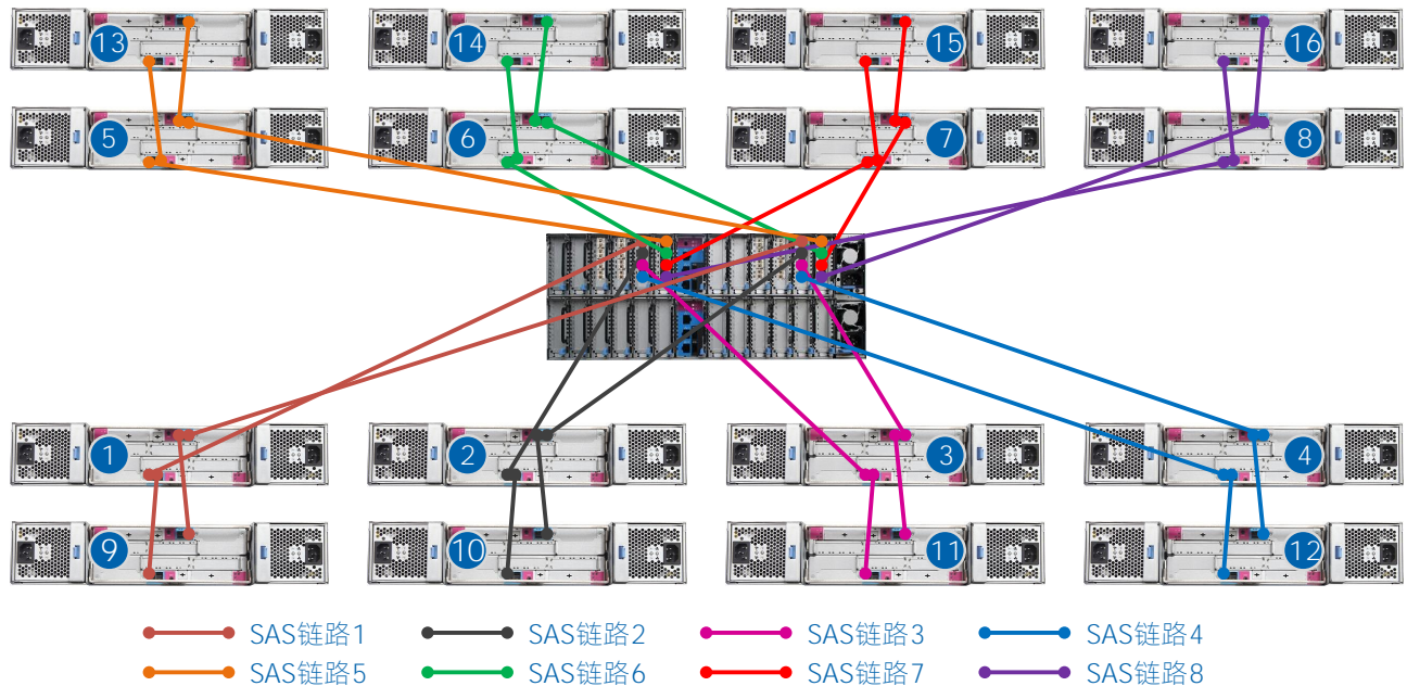
图 5-2 连接 16 台扩展柜（每控 2 张 4 口 SAS 卡）
