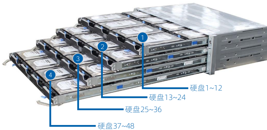
图 3-4 3U 扩展柜硬盘模块结构图
