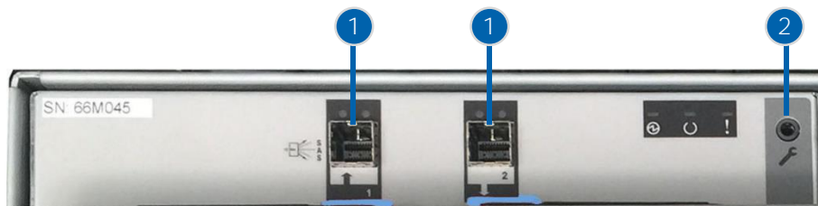
图 3-13 ESM 模块后视图
