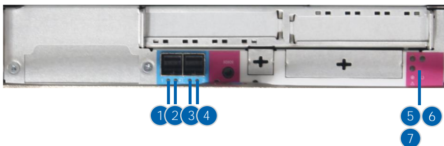
图 4-12 2U/3U 扩展柜 IO 模块指示灯
