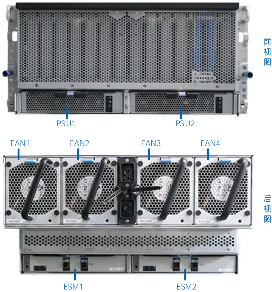
图 3-6 5U 扩展柜前后图
